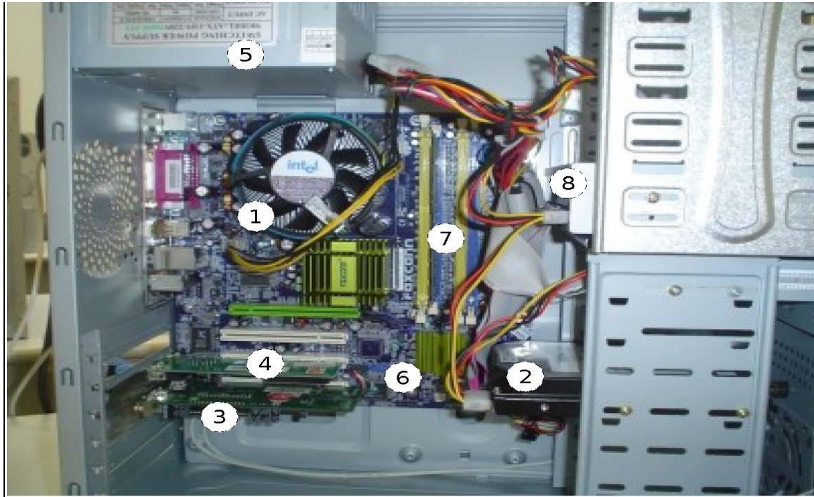
(1) processador, (2) disco rígido, (3) placa de vídeo, (4) placa de rede, (5) fonte de energia, (6) placa-mãe, (7) módulos de memória, (8) leitor de CDs.
